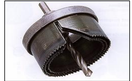
26.105.02 9002648011098 Apvalių grąžtų medžiui rink. PROFI KAUFMANN;h–52mm;d–60-67-74mm
